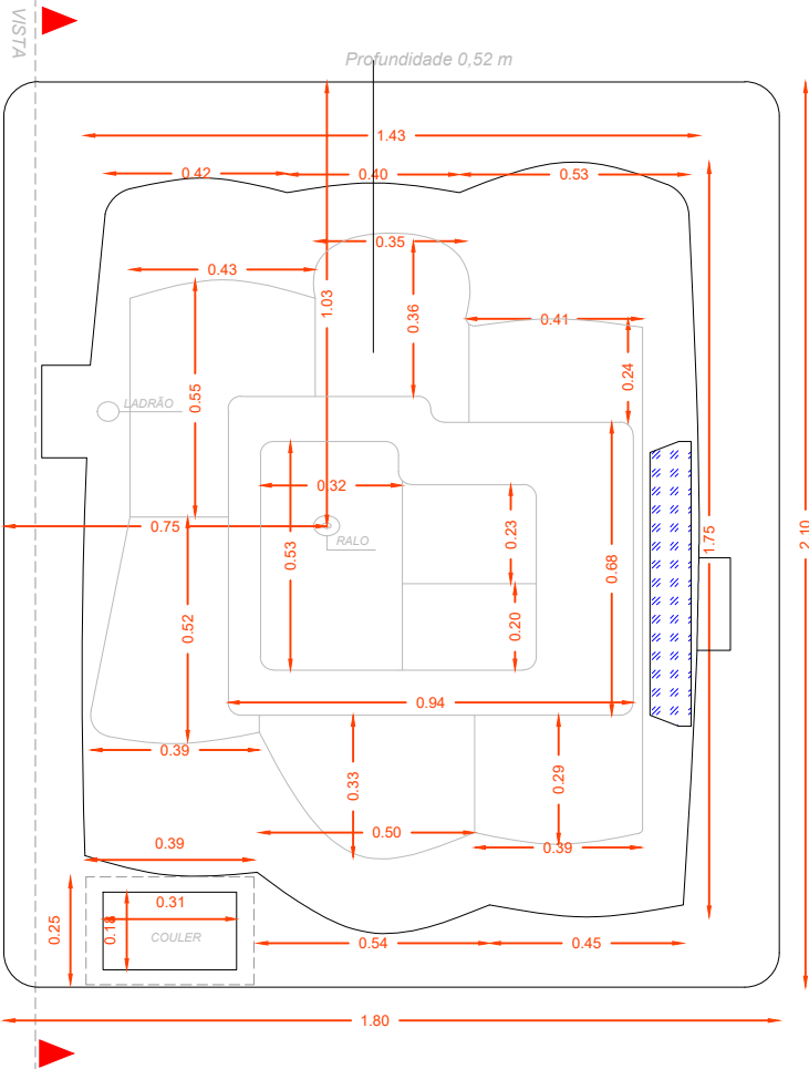
PLANTA BAIXA DIMENSÕES EM : METROS
