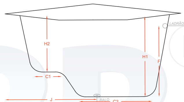
VISTA LATERAL
